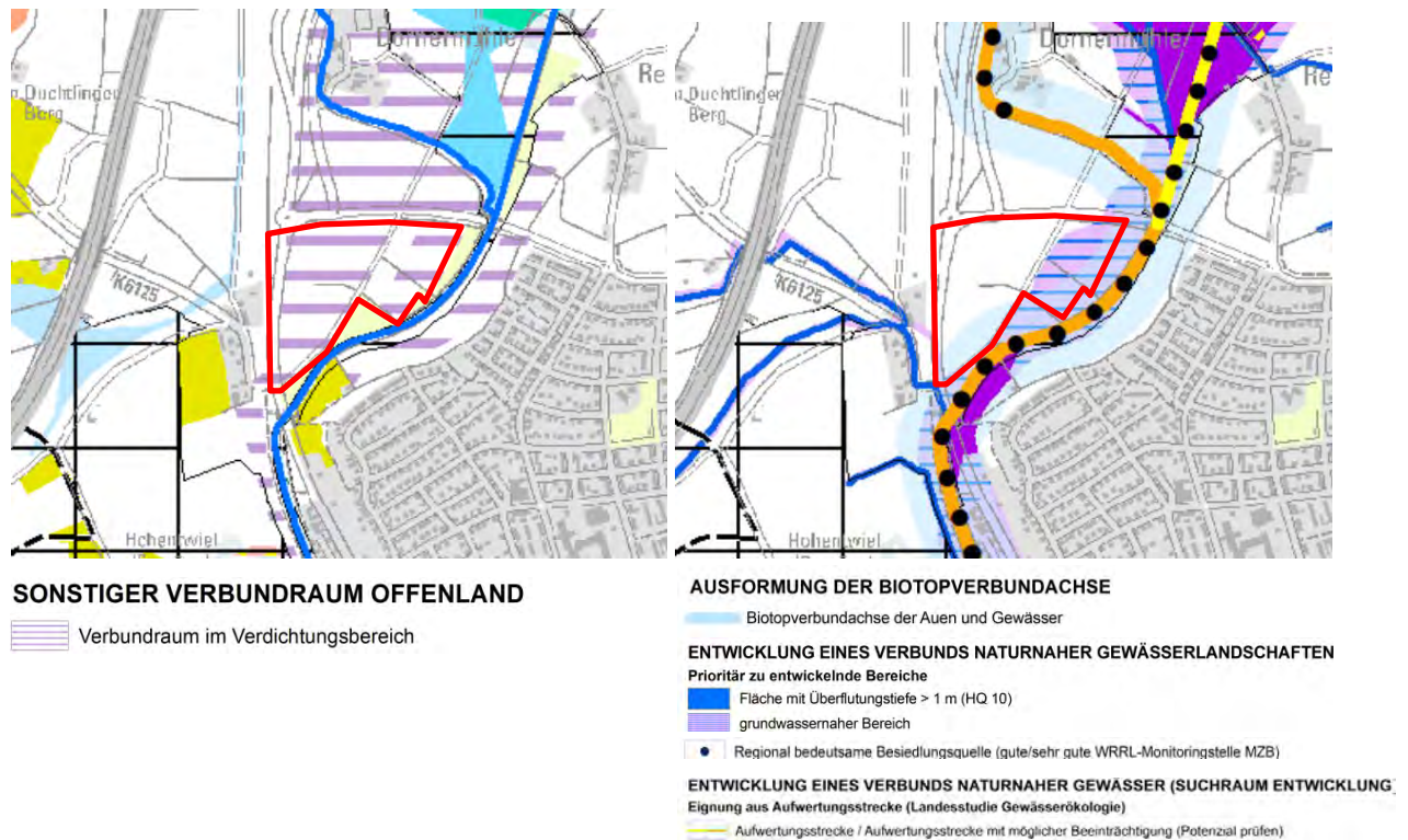
Abb. 7: Regionaler Biotopverbund des Regionalplans Hochrhein-Bodensee, Offenland (links), Gewässer (rechts) unmaßstäblich, Plangebiet: rot
