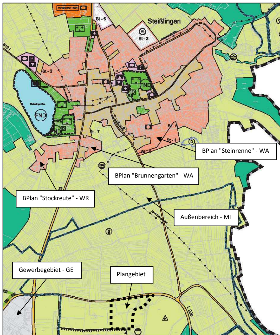
Abbildung 1 - Gebietseinstufung
