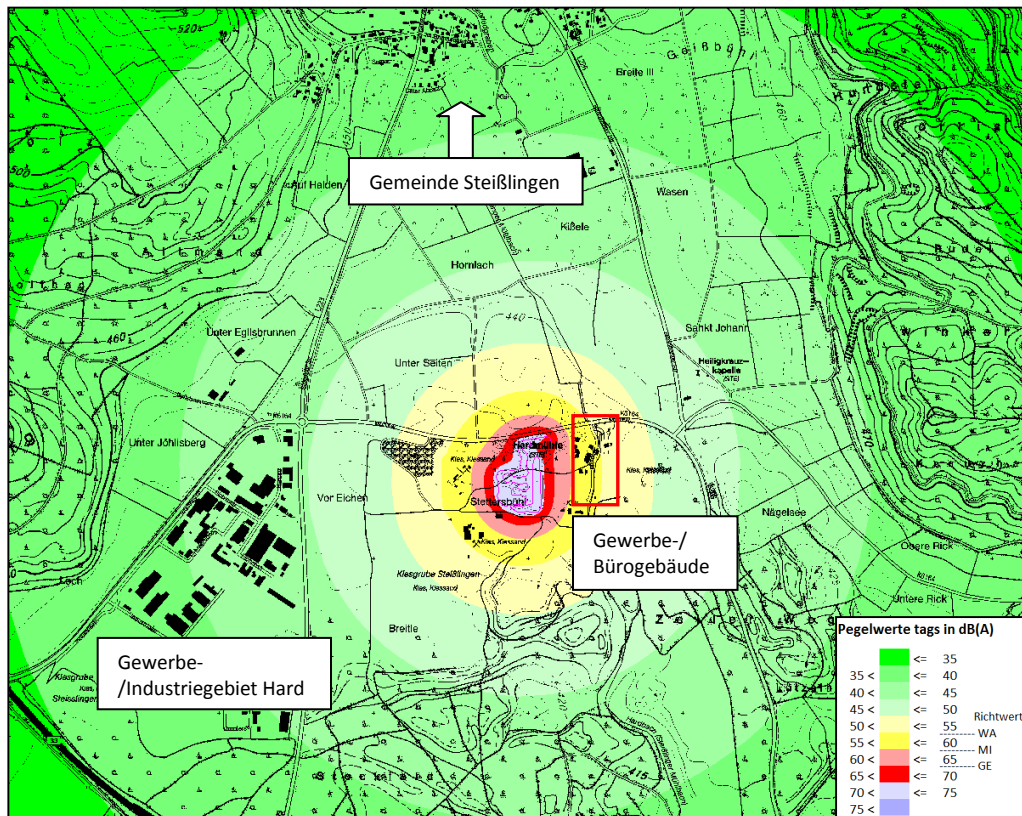
Abbildung 5 - Wettbewerbsbetrieb -tags
