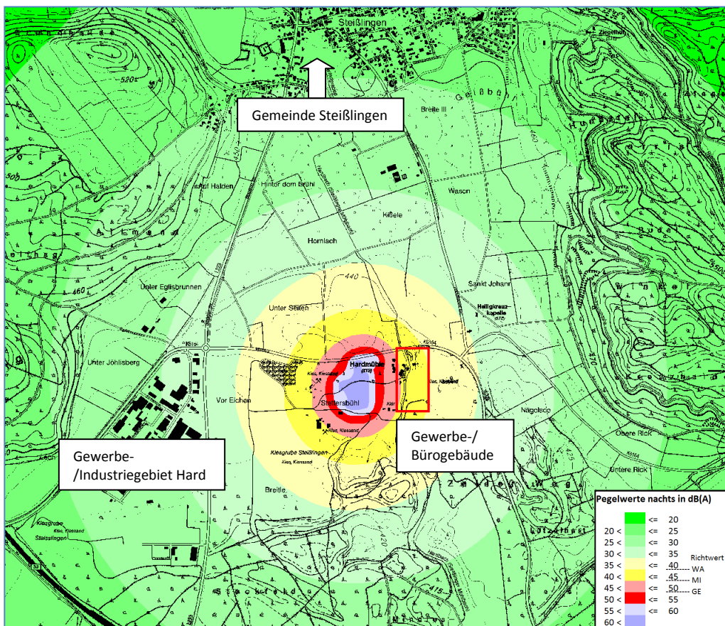
Abbildung 4 - Trainingsbetrieb - nachts
